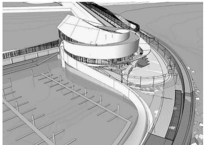
Figura 38. Bacia de rotação de autocarros e do eléctrico do lado sul do edifício.
