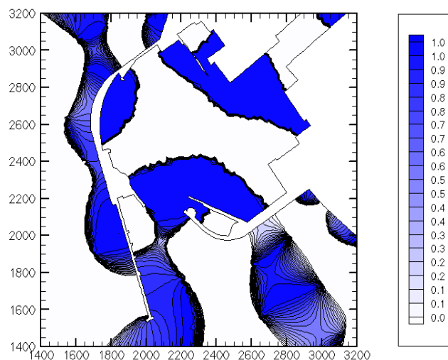
Figura 28. Estudo das condições de ressonância no interior do porto de Leixões. Diagrama de fase de onda. Nível de maré igual a 2 m ZHL, período de onda de 70 s e rumo local igual a 27°, IHRH (2007).
