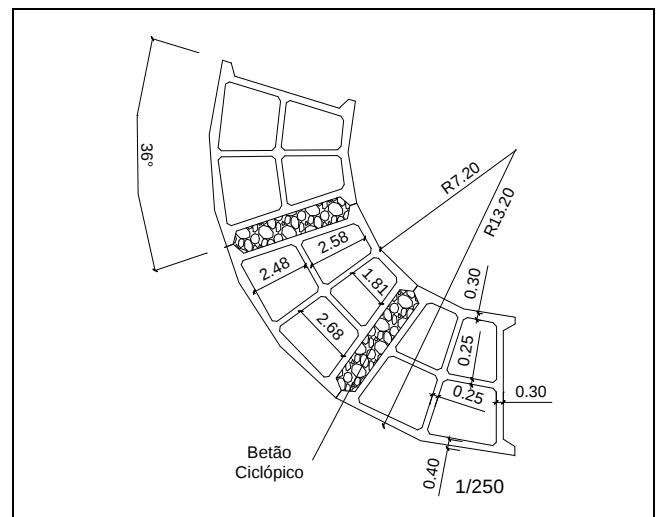
Figura 24. Pormenor da ligação entre aduelas, IHRH (2006).
