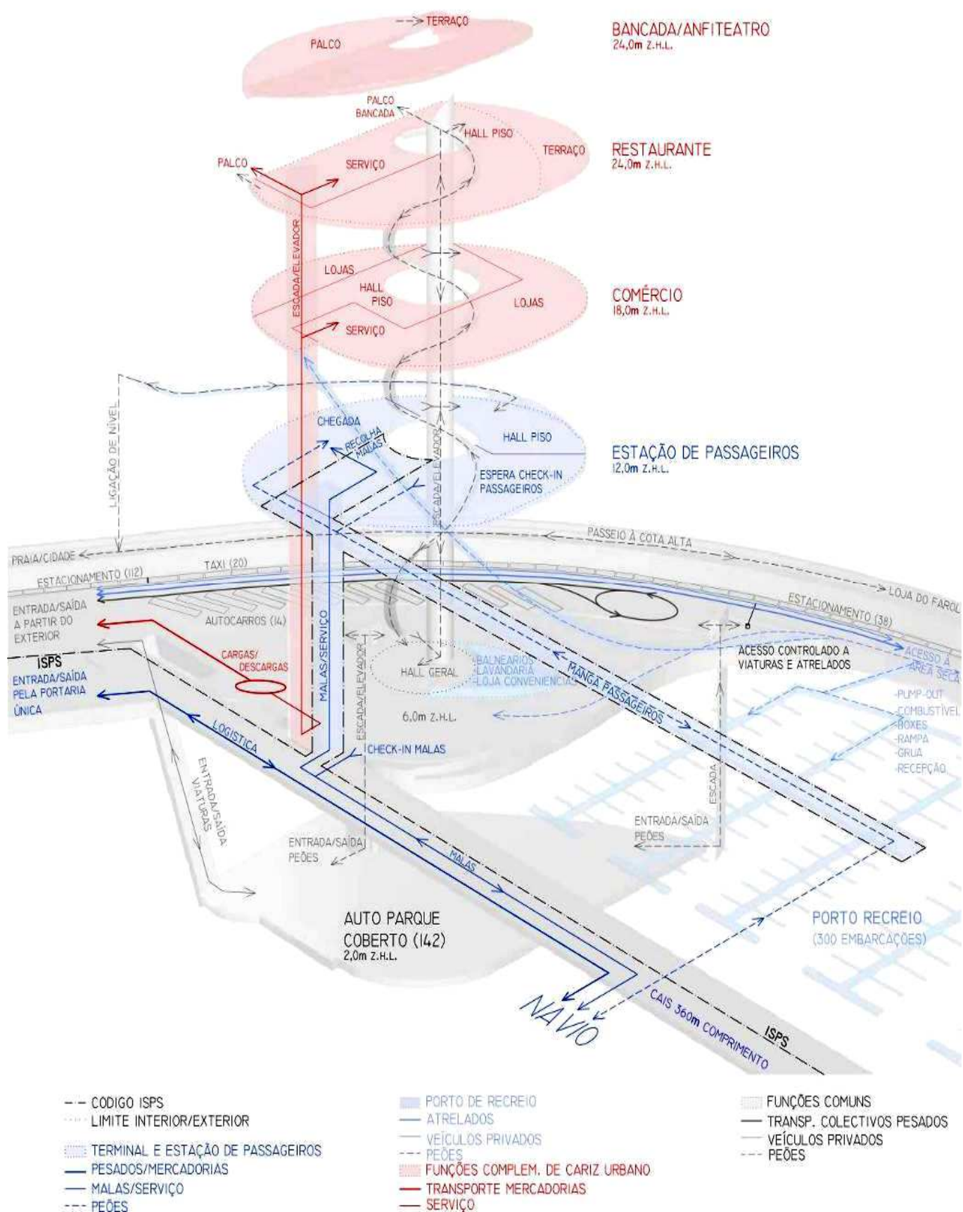
Figura 2. Interligação entre as diferentes funções e espaços associados ao projecto.
