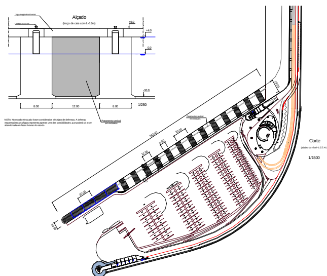
Figura 26. Layout do projecto correspondente à fase de revisão do Estudo Prévio, IHRH (2007).
