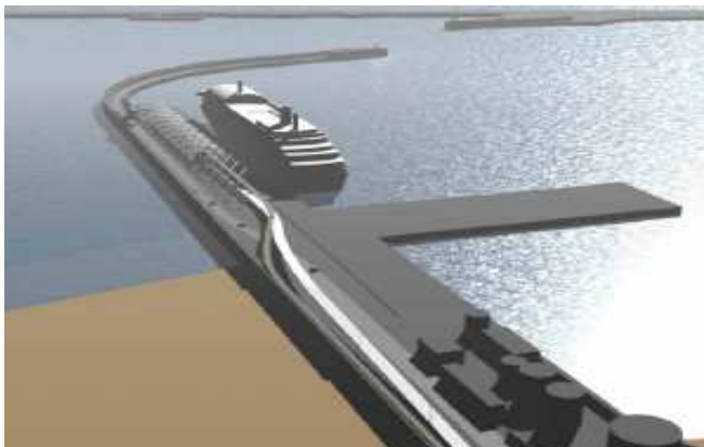
Figura 17. Cenário “B” estudado na 2.ª fase do Estudo Prévio.
