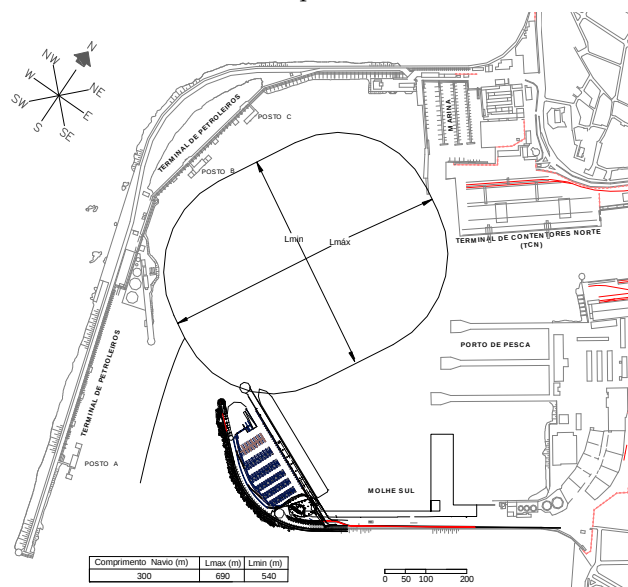
Figura 25. Bacia de manobra de um navio de cruzeiro com 300 m de comprimento. Identificação de zonas de risco de conflito com outras actividades portuárias, IHRH (2006).
